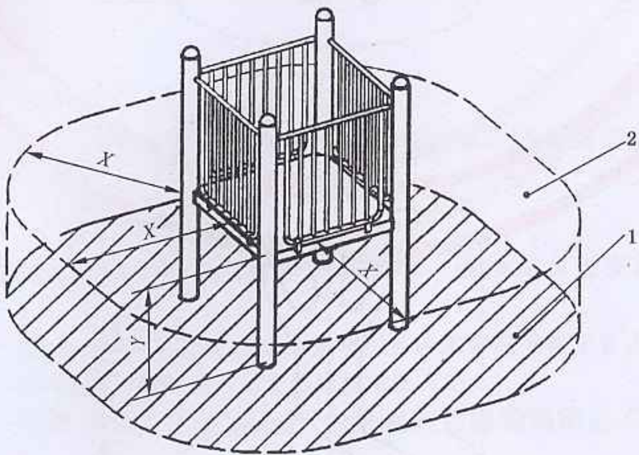
图 13 碰撞区域尺寸范围
