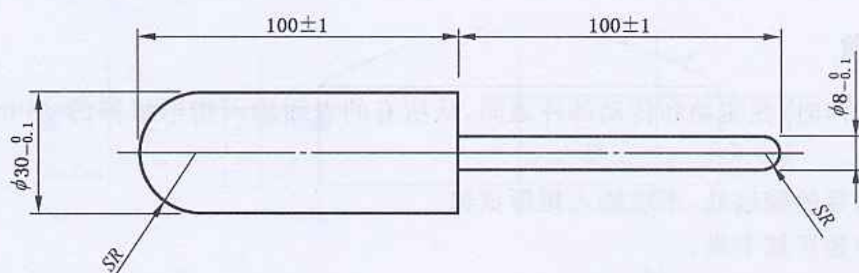
图 37 指形试棒
