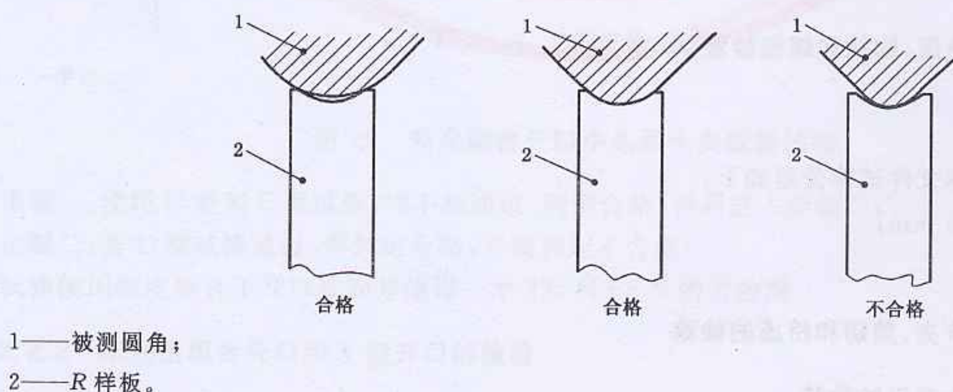
图 26 圆角测量
