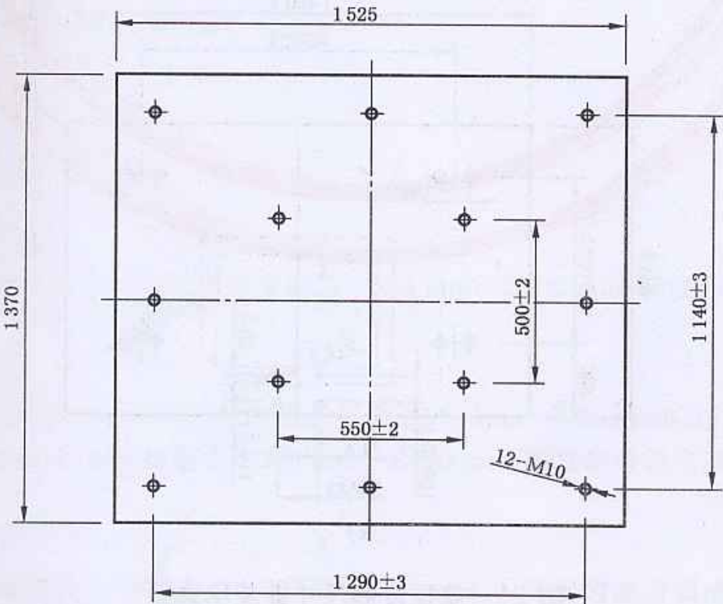
图 22 乒乓球台面背部安装尺寸示意图
