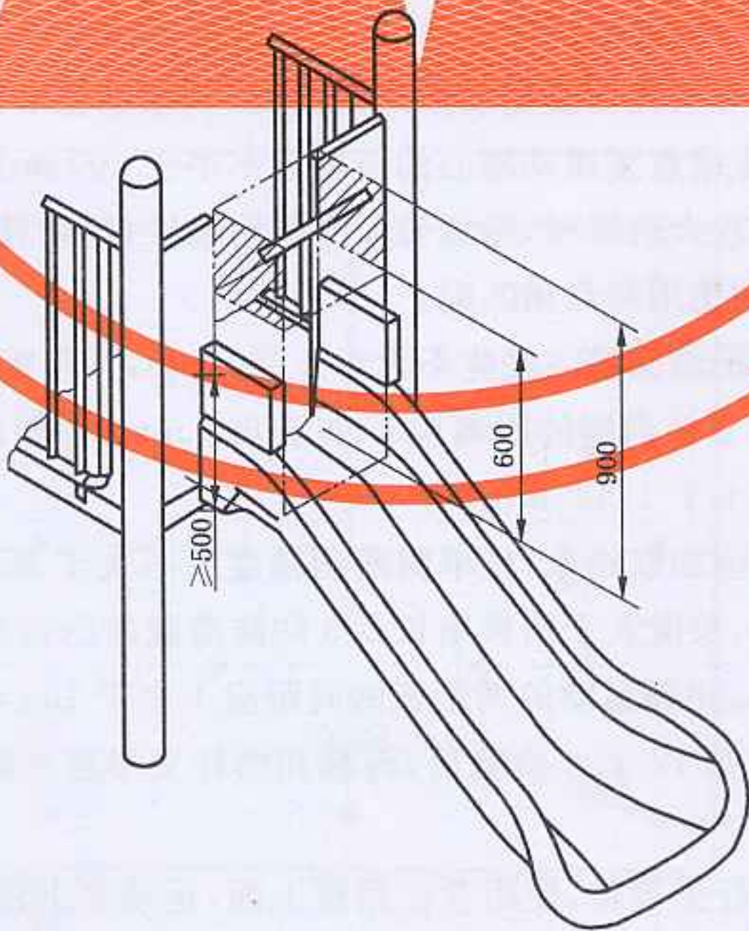
图 23 起始区的侧面防护和栏杆的示例
