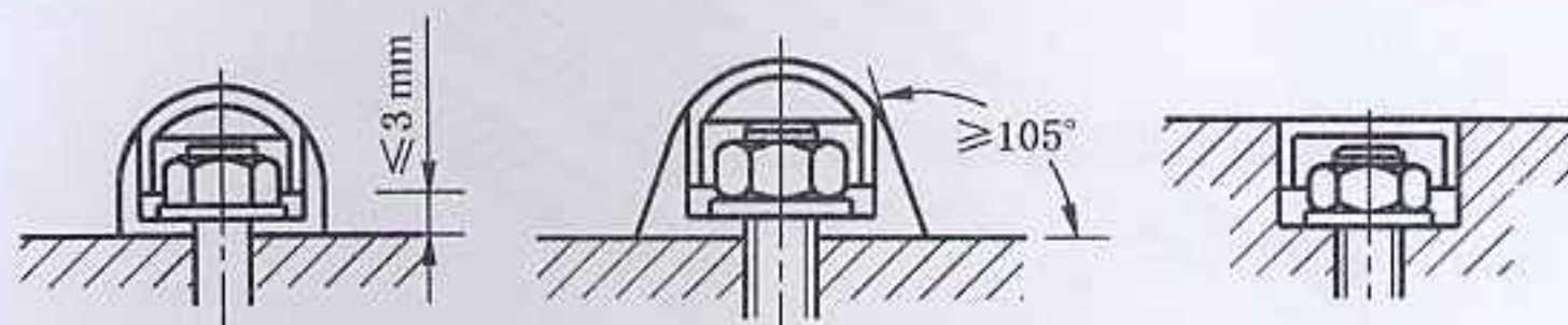
图 7 螺栓防护
