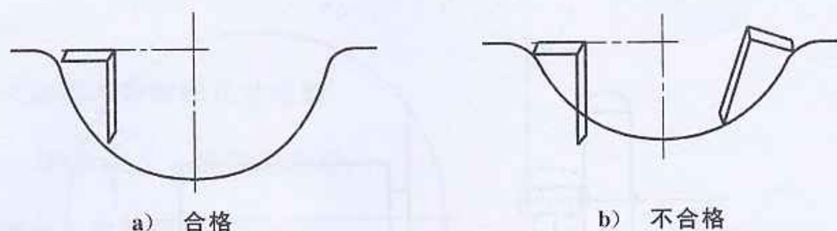
图 49 滑行区轮廓检验
