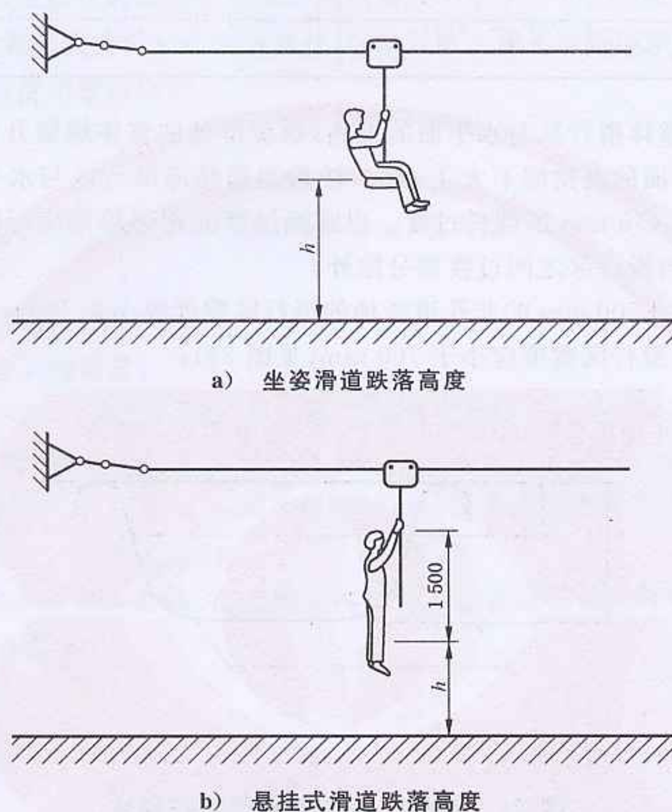
图 25 悬垂类滑道图示
