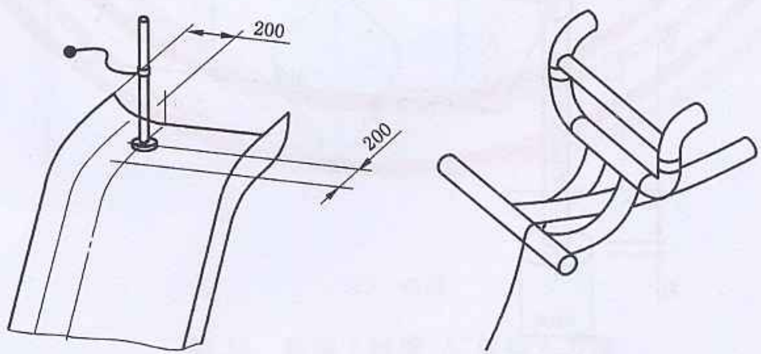
图 36 钩挂检验示例
