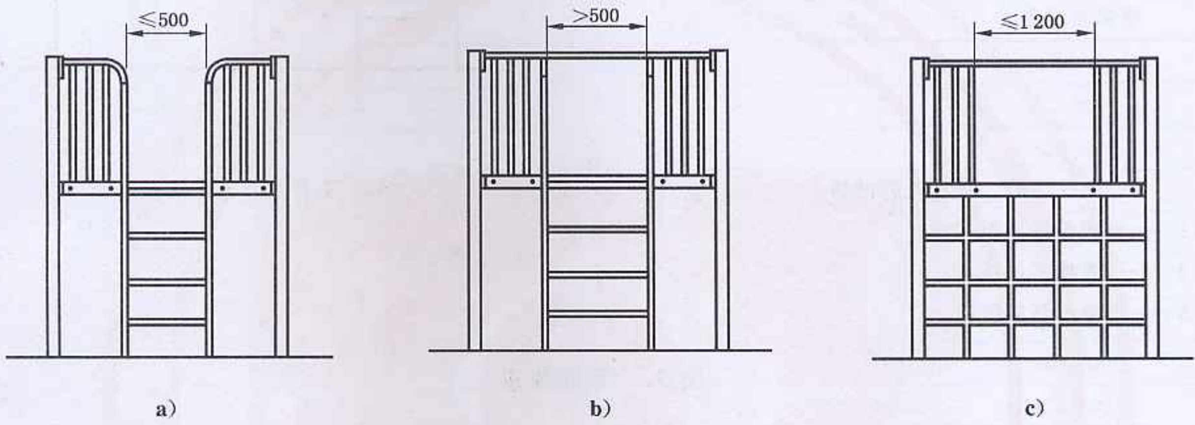
图 19 栅栏出入口
