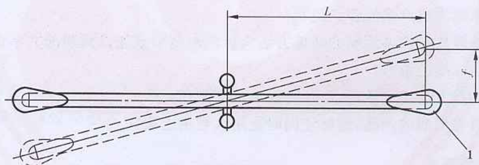
图 46 冲击试验变形测量
