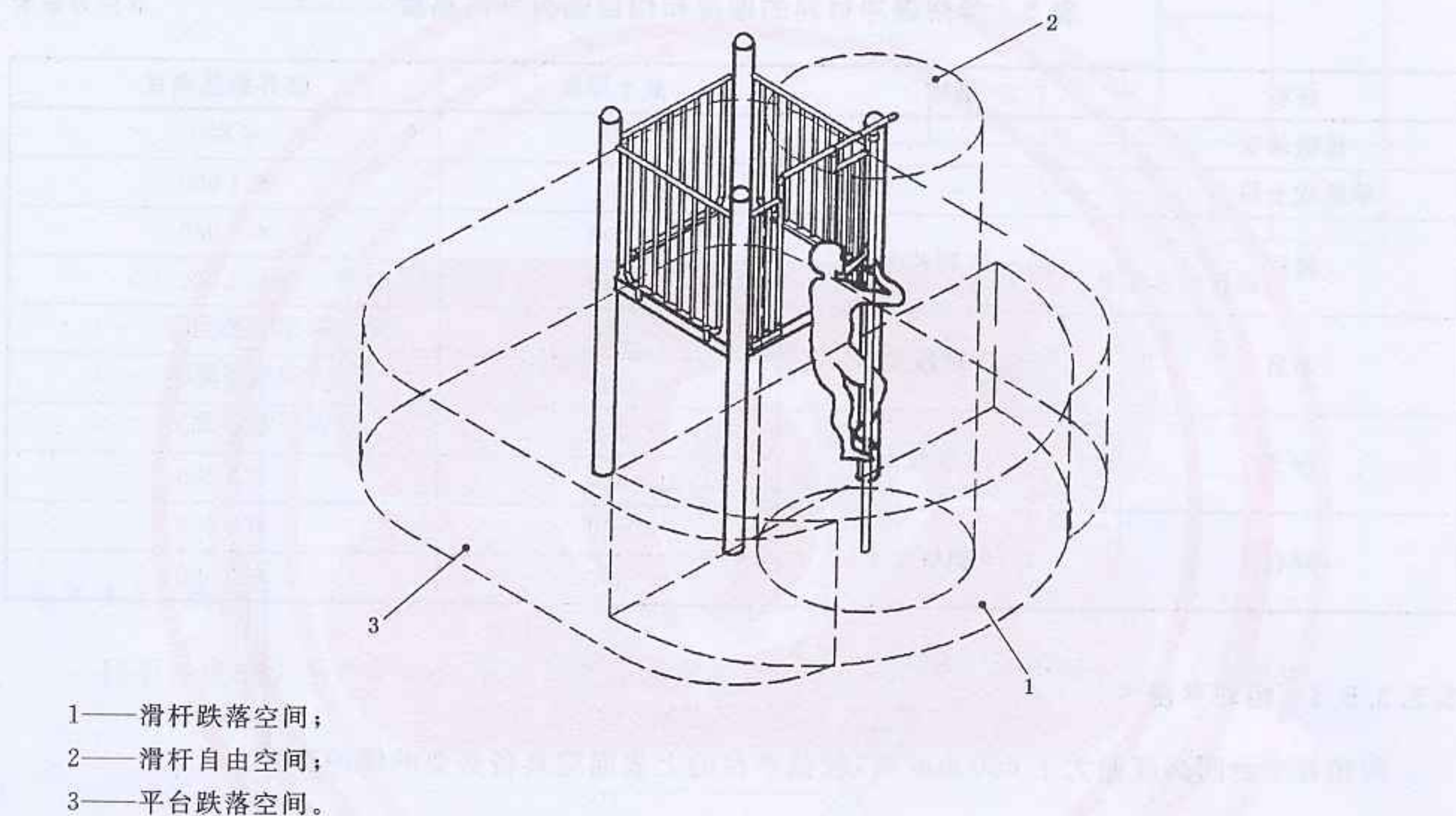
图 15 滑杆跌落空间与自由空间
